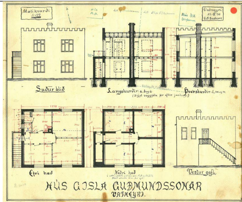
Mynd 22. Uppdráttur Gests Ó. Gestssonar byggingarmeistara af Strandgötu 13. (Teikningasafn b.fulltrúa Vesturbyggðar.)
